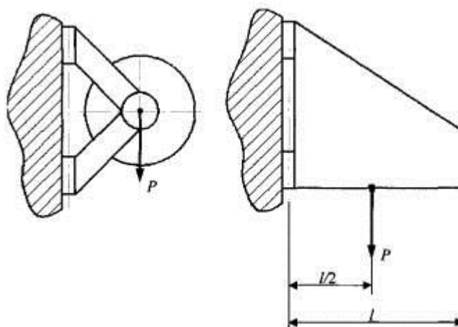
Рисунок 1 - Схема приложения нагрузки P к рукавной кассете
